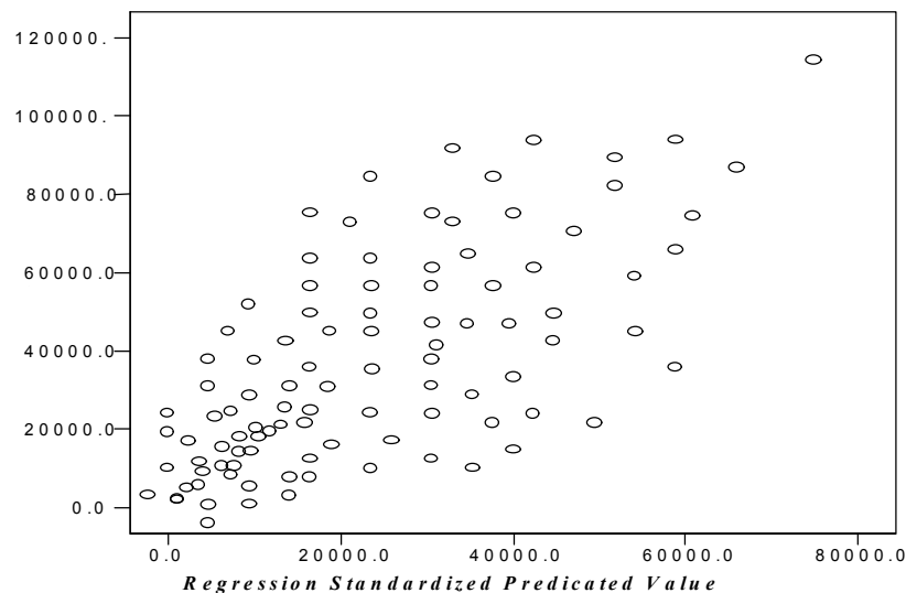
Gambar.3 Output Hasil Uji Heteroskedastisitas dengan Scatterplot Dependent Variabel : Nilai Produksi
