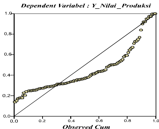
Gambar.2 Output Hasil Uji Normalitas dengan Normal P-Plot Normal P-Plot of Regression Standardized Residual
