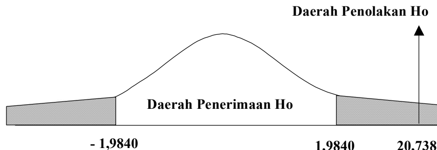
Gambar 6 Pengujian hipotesis antara biaya bahan baku Secara parsial terhadap nilai produksi
