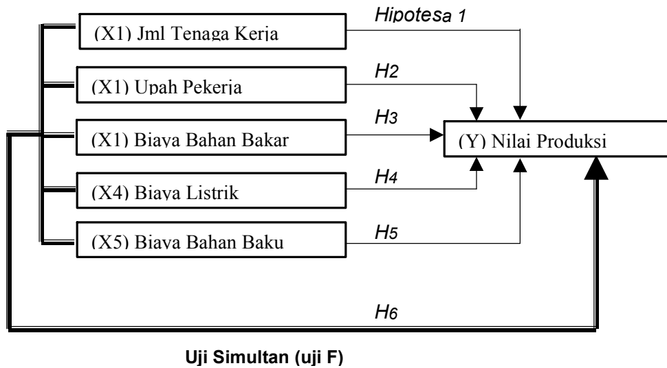
Gambar .1 Path Diagram Kerangka pemikiran
