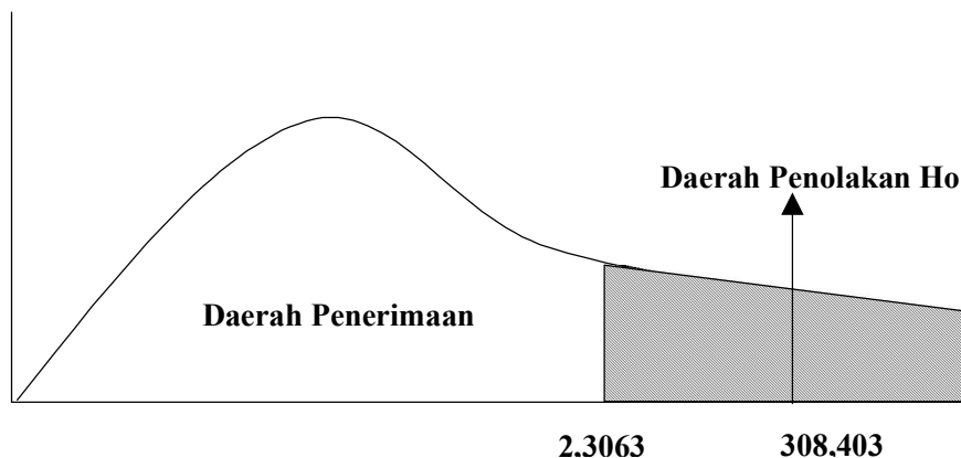
Gambar 5 Pengujian hipotesis kelima variabel bebas (Xi) Secara Simultan
